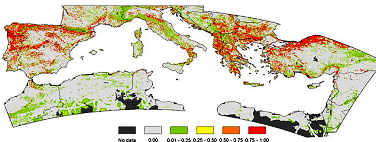
Рисунок 7. Оценка RLA для стран средиземноморского бассейна (Weissteiner et al., 2011)
