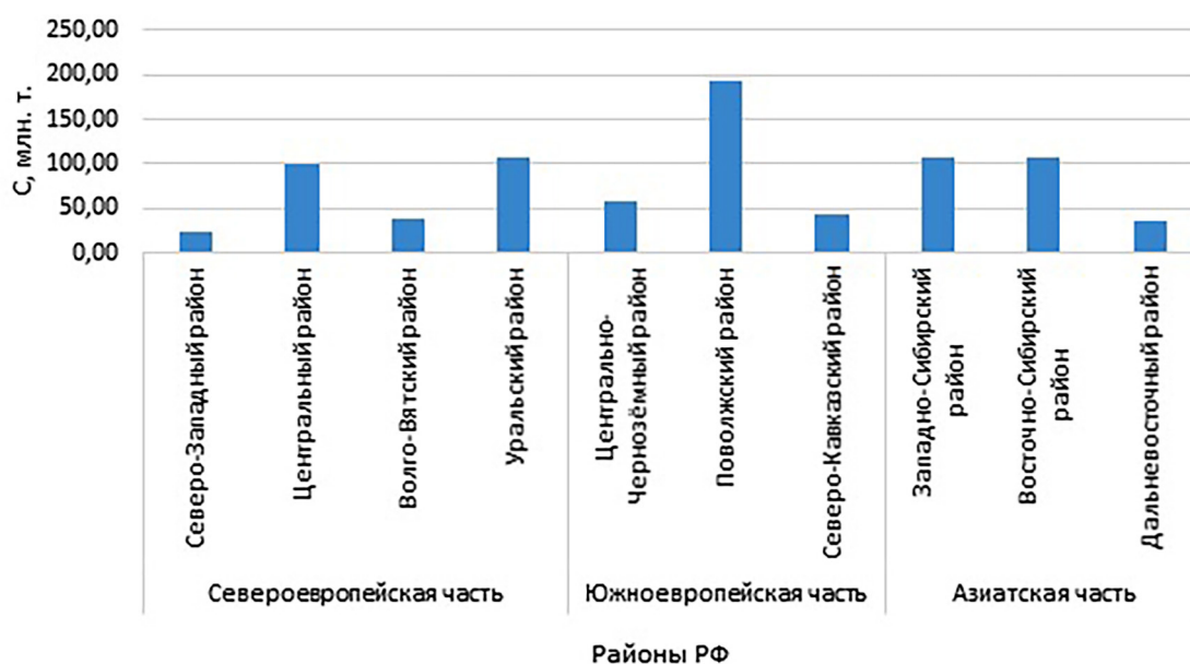
Рисунок 6. Депонирование углерода в двадцатисантиметровом слое почвы заброшенных с.-х. земель в период с 1990 по 2009 гг. (по: Kurganova et al., 2014)
